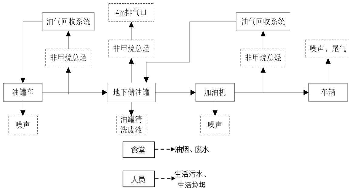
图 2-2 项目工艺流程及产污节点图
